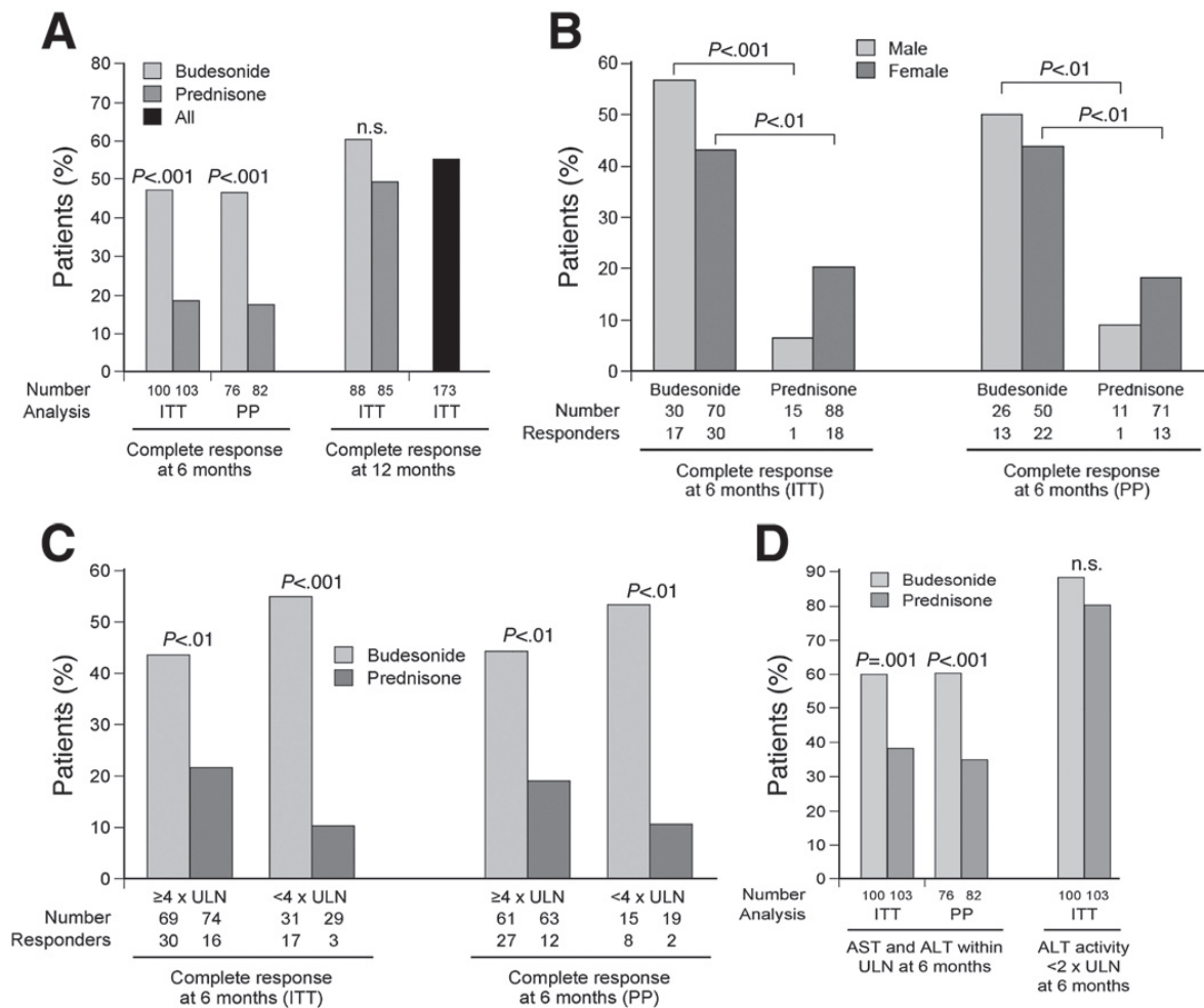
Рис. 2. А – достижение полной ремиссии для ИТТ-популяции и РР-популяции; В – достижение полной ремиссии в зависимости от пола; С – достижение полной ремиссии к 6-му месяцу терапии по сравнению с исходным уровнем аминотрансфераз; D – достижение полной биохимической ремиссии к 6-му месяцу терапии по сравнению с биохимической ремиссией (уровень АЛТ < 2 норм к 6-му месяцу).
