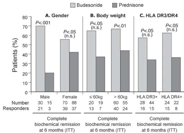
Рис. 3. Достижение полной биохимической ремиссии в зависимости от пола (А), массы тела (В), антигена HLA (С).
